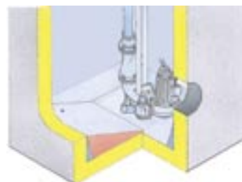
Stroomprofiel éénpompsuitvoering.
