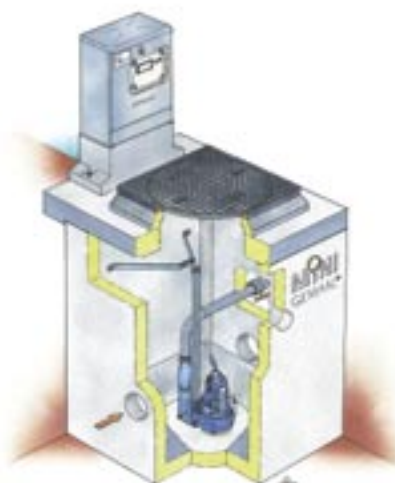
Het Minigemaal
