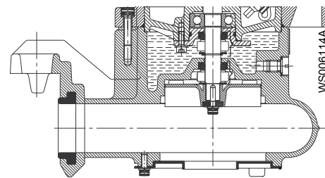
Afbeelding 8: D-waaier
