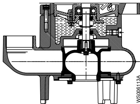
Afbeelding 7: C-waaier
