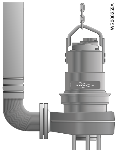
Afbeelding 4: F-installatie
