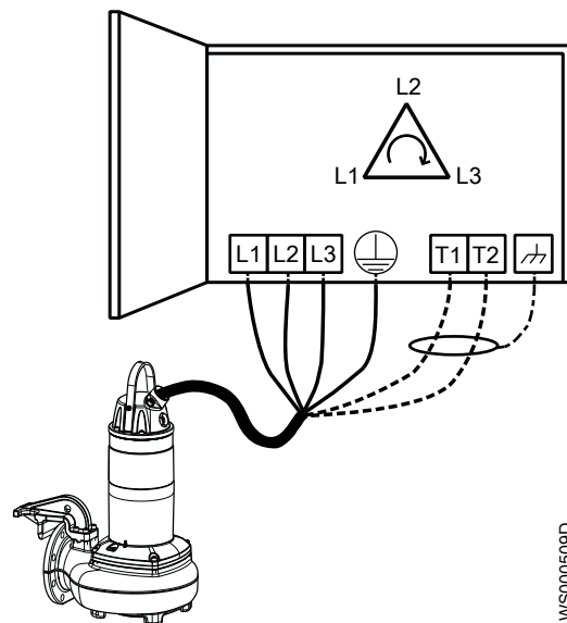
Afbeelding 6: Fasesequentie
