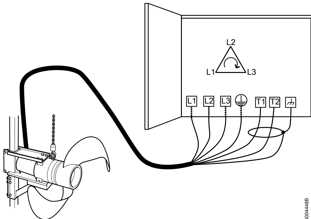
Afbeelding 4: Aansluiting van de motorkabel.
