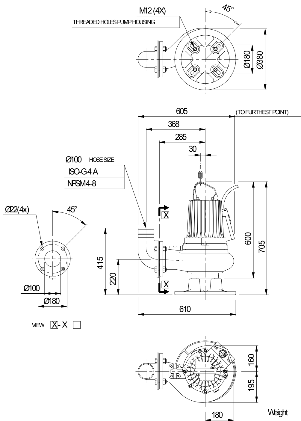
Dimensional dwg CS3102MT
