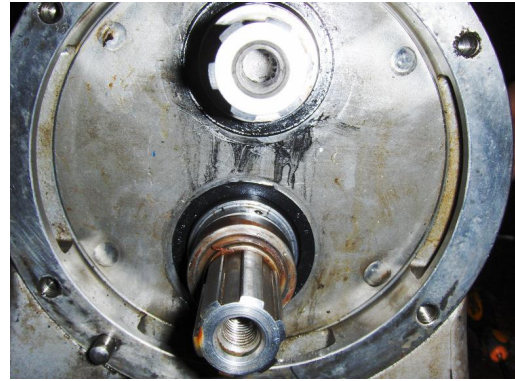
Olie lekkage langs de as en keerring
