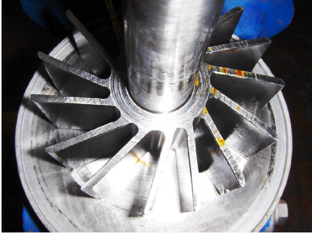
Smalle schoepenwiel met aanloopschade
