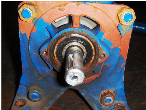
Lager met roest A.Z.
