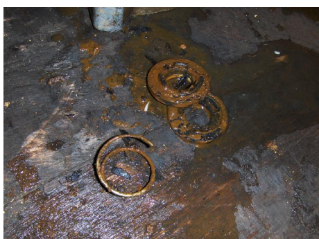
Mechanical Seal volledig stuk gedraaid.
