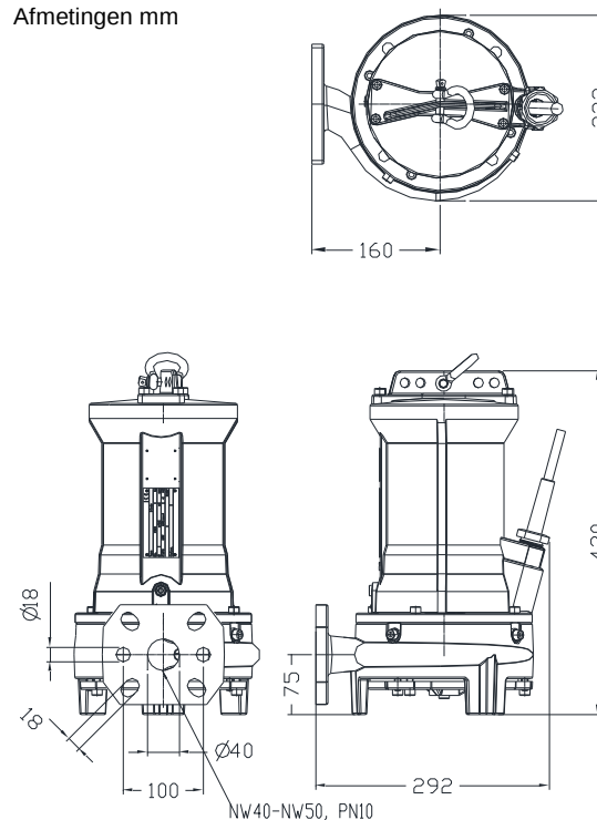
Afmetingen mm
